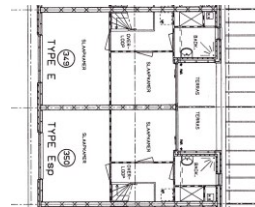
plattegrond 5e verdieping
