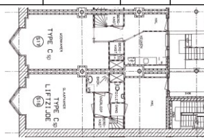
plattegrond 1 e verdieping
