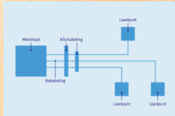
Schema van stervariant
